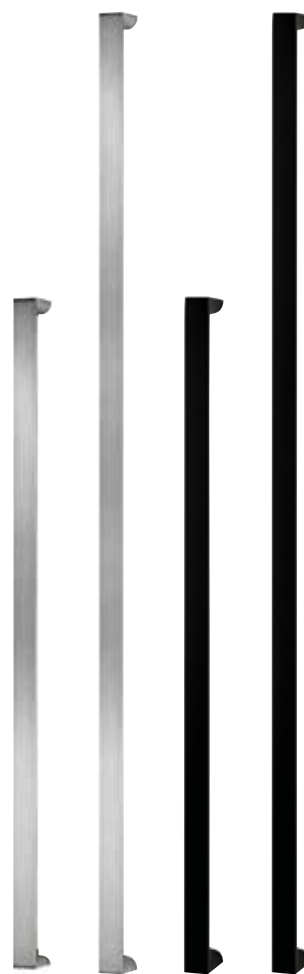
Griffstange halbrund Edelstahl matt gebürstet oder Schwarz Finea 370 mit geraden Stützen HA 312 Länge 1.040 mm HA 289 Länge 1.480 mm
